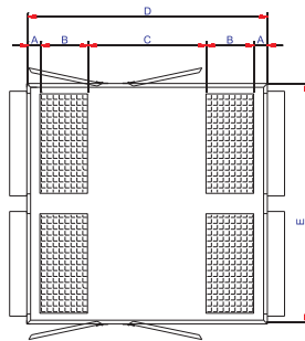
Onderaanzicht
