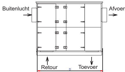
Vooranzicht
