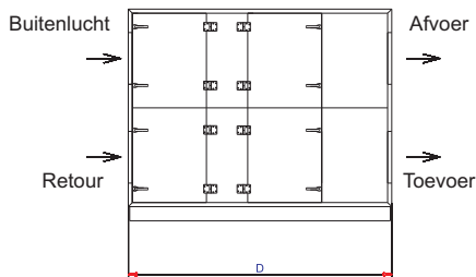
Vooranzicht
