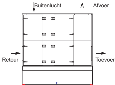
Vooranzicht
